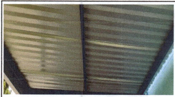
FOTO 10: Sustitución de lámina, por lámina troquelada aluzinc calibre 26 PATIO II
